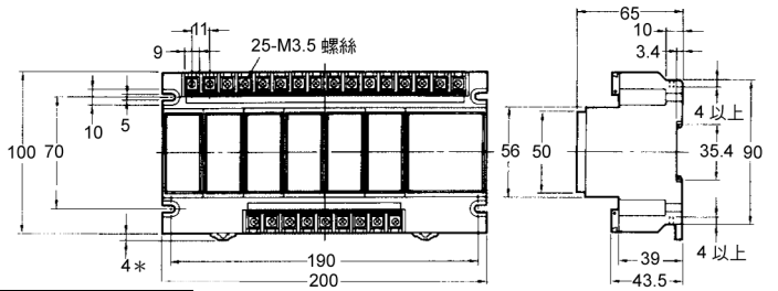
CAD 檔 61F-09 *DIN 鋁軌安裝插入 slider 時的尺寸
