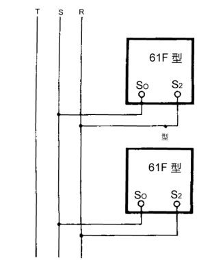
圖 2：電源相位一致
