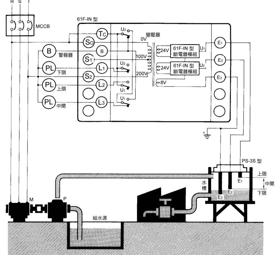
繼電器配置
