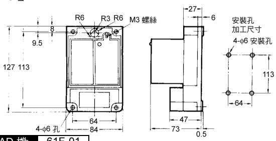
CAD 檔 61F-01
