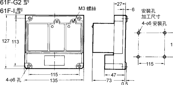
CAD 檔 61F-02
